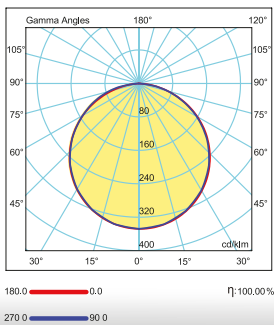
FOTOMETRİK EĞRİ
