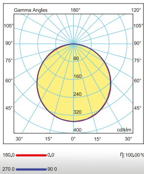
FOTOMETRİK EĞRİ
